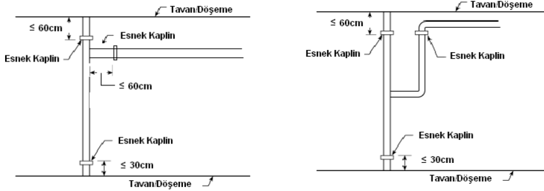
Şekil 9.5.2.3 Çok katlı binalarda esnek kaplin yerleşimi
