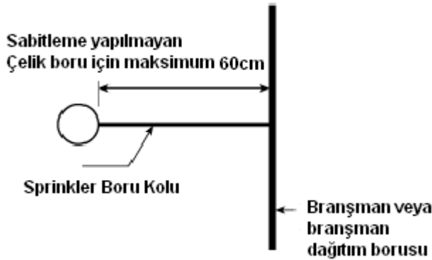
Şekil 9.4.1.6(a) Sabitleme yapılmayan boru kolu mesafesi
