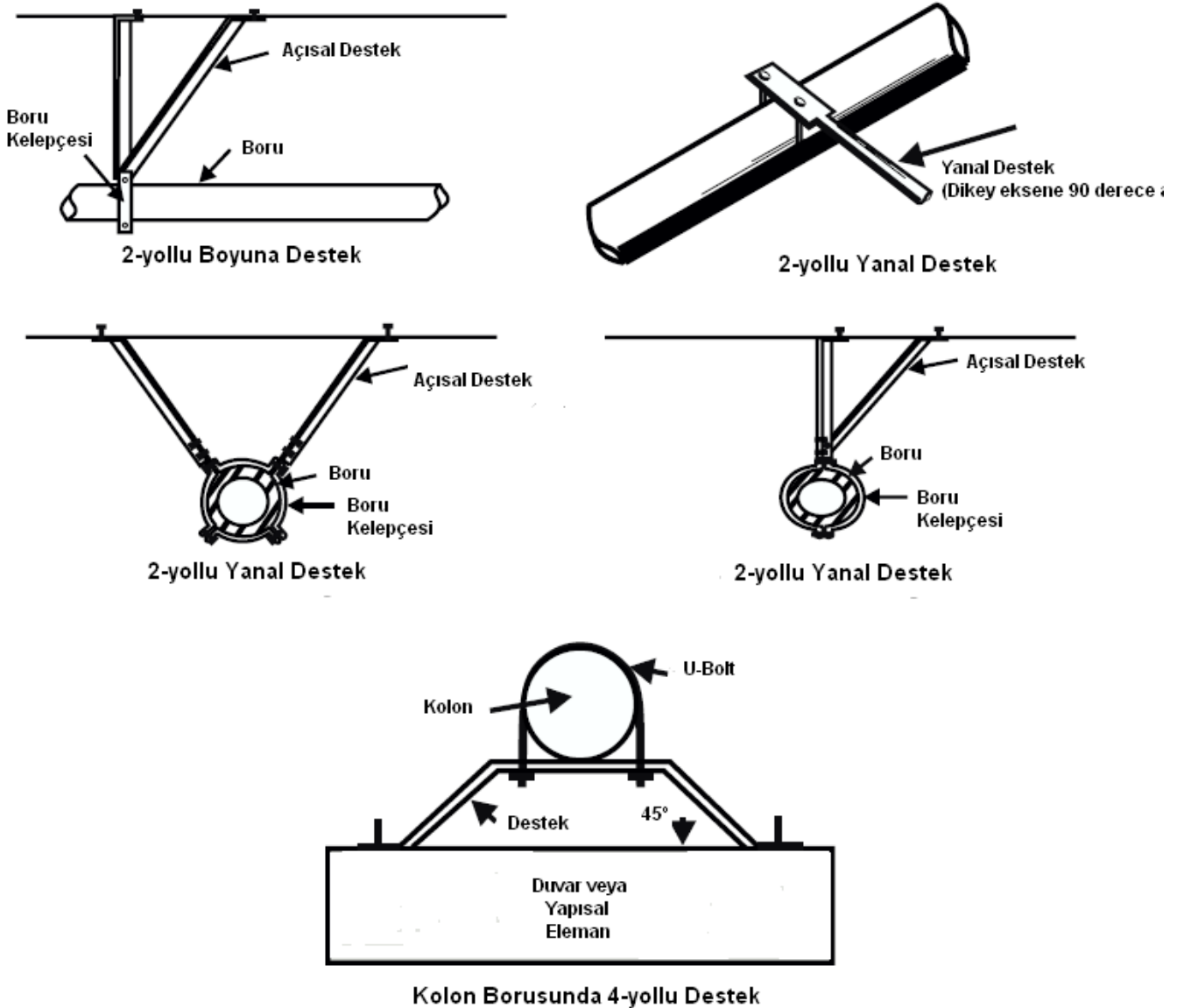
Şekil 9.5.4 Deprem Destek Tipleri
