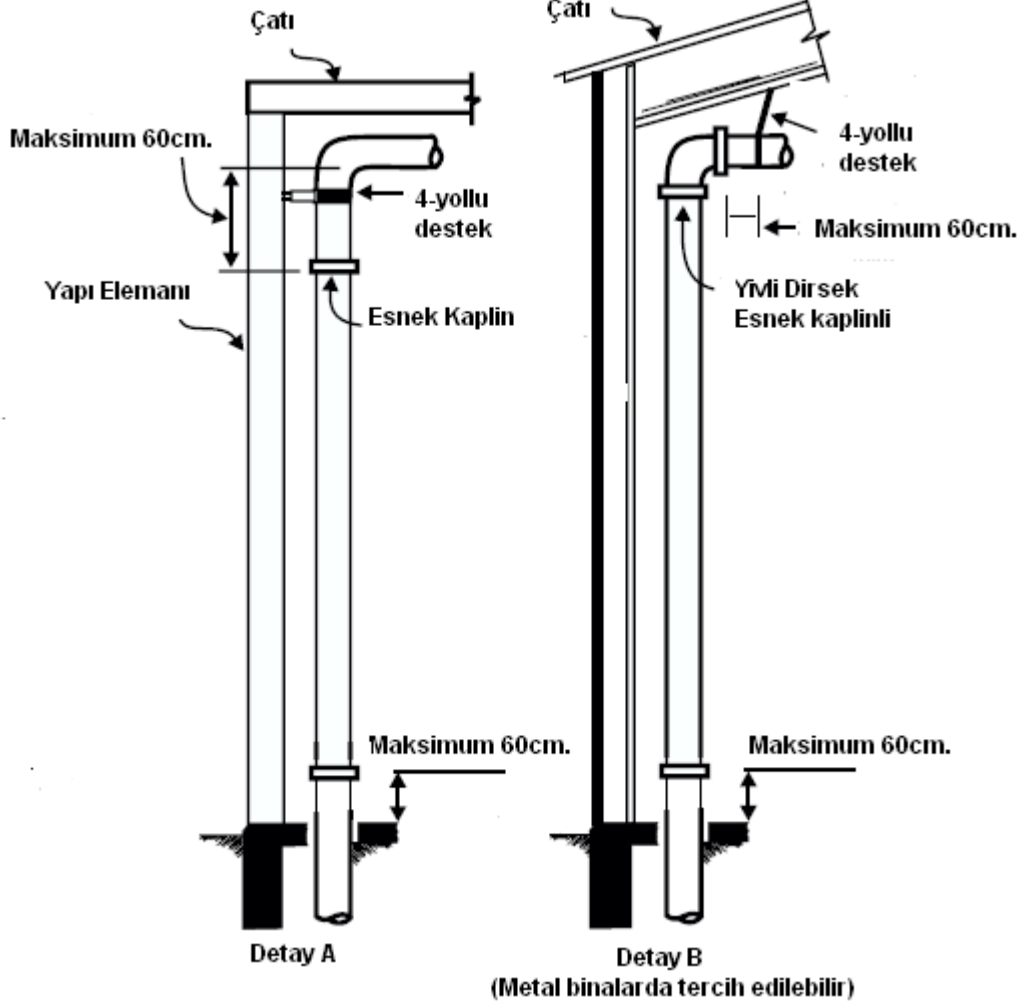
Şekil 9.5.5.1(a) 4 yollu destek yerleşimi
