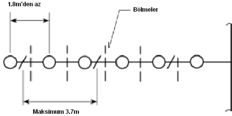
Şekil 9.5.1.1(b) Askılar arası mesafeler
