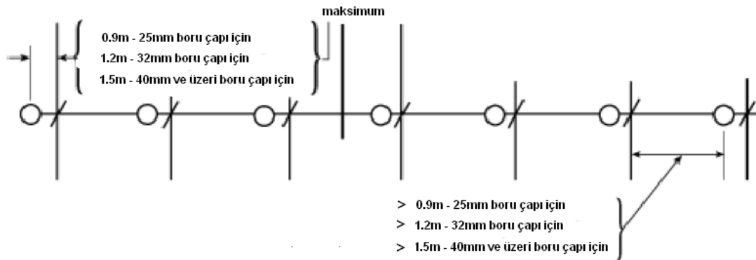
Şekil 9.4.1.5(a) En son sprinklerin boru askılarına mesafesi
