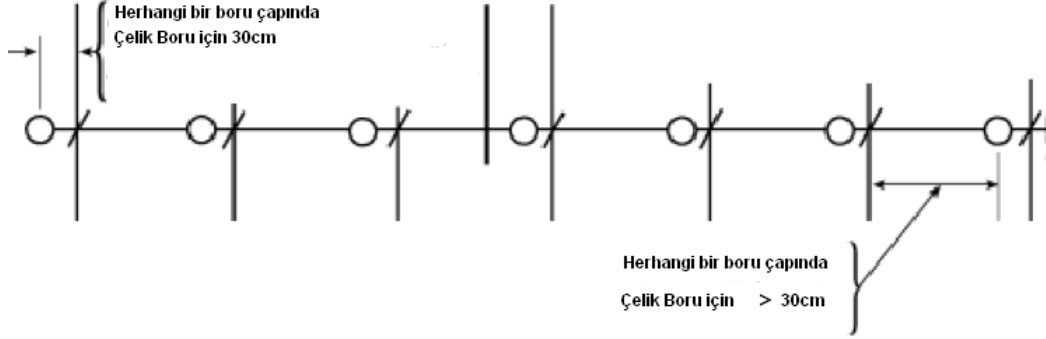
Şekil 9.4.1.5(b) En son sprinklerin boru askılarına mesafesi
