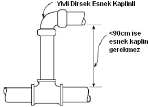
Şekil 9.5.2.2 Kolon borularında esnek kaplin yerleşimi
