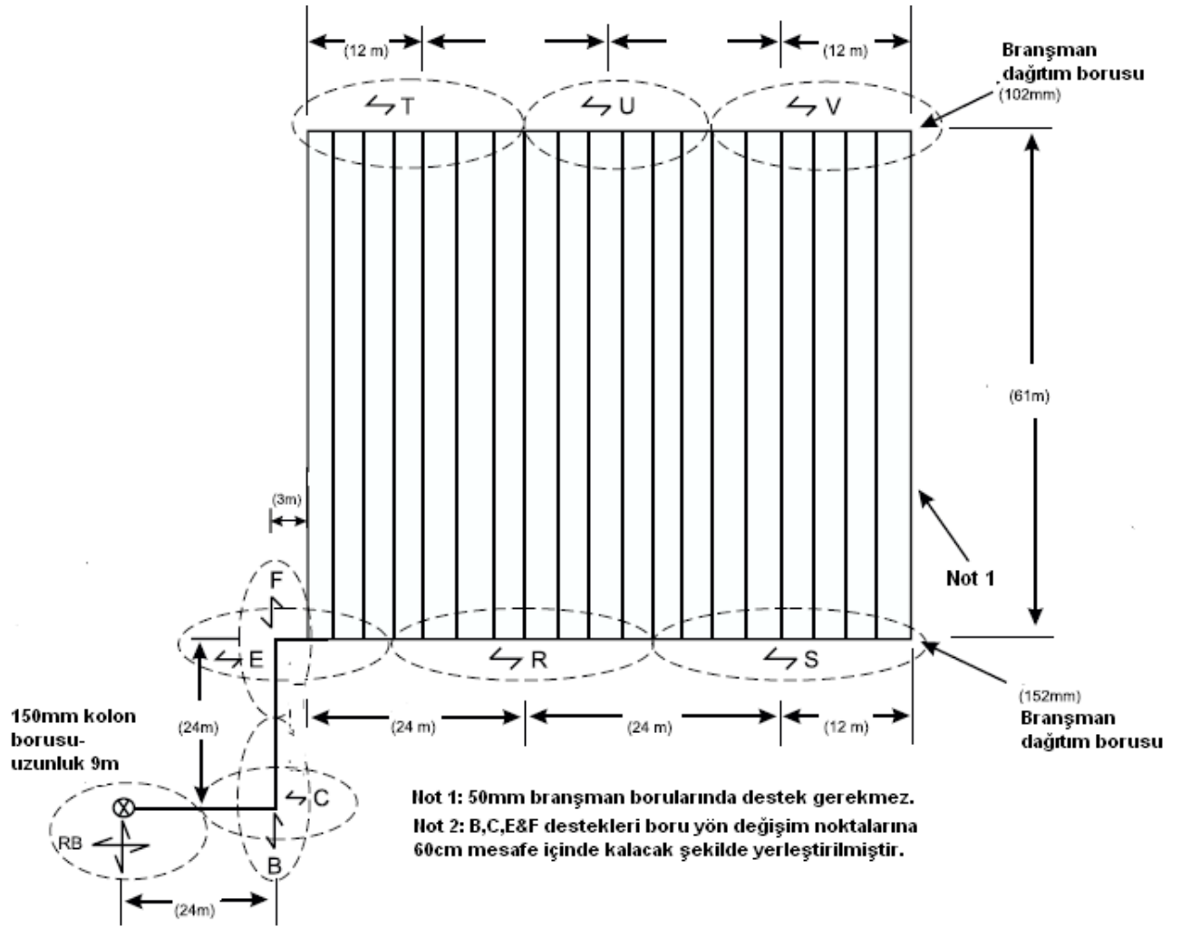
Şekil 9.5.6.1(b) Örnek: 2-yollu boyuna destek ve 4-yollu desteklerin etkileme zonları
