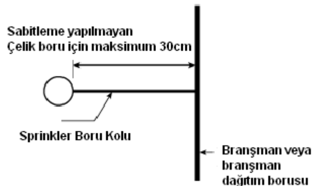
Şekil 9.4.1.6(b) Sabitleme yapılmayan boru kolu mesafesi (P&gt;6.9bar)
