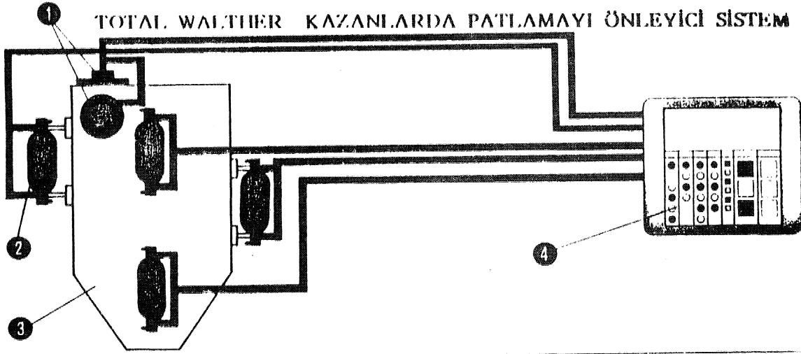
1. Patlama dedektörü 2. Söndürücü haznesi 3. Kazan 4. Kontrol paneli
