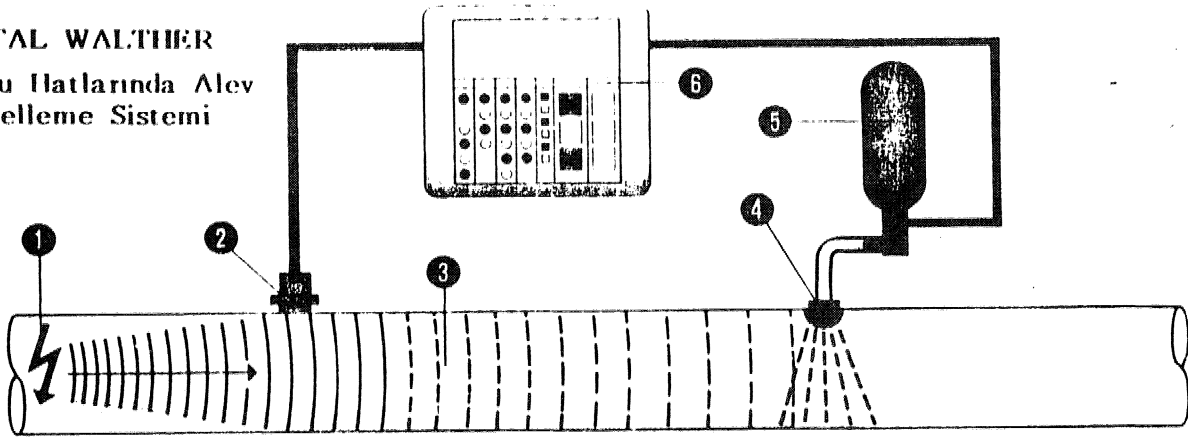
1. Kivılcım 2. Infrared dedektörü 3. Alev sonrası 4. Nozül 5. Söndürücü haznesi 6. Kontrol paneli
